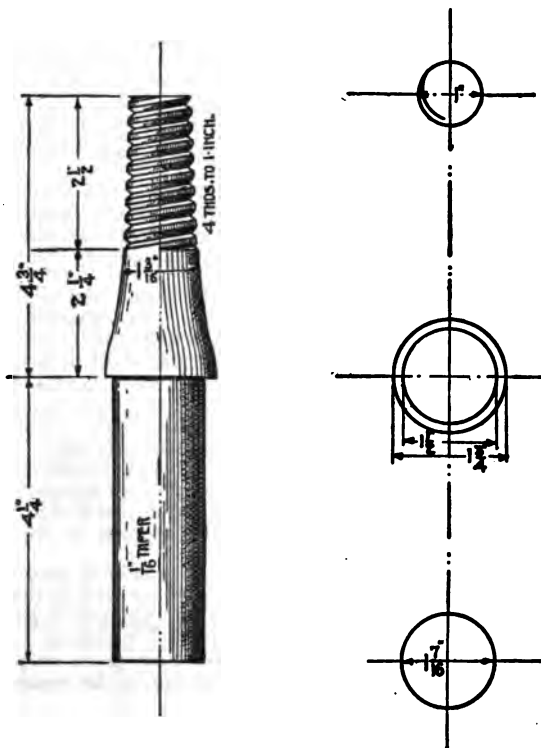
FIG. 92.—Standard N. E. L. A. wood pin.
