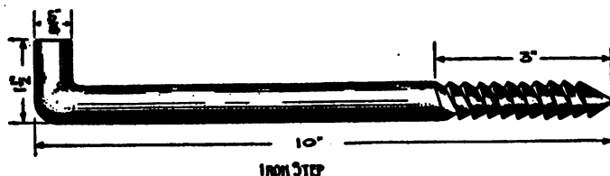
FIG. 109.—Standard pole step.
