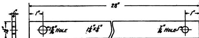
FIG. 107. Standard N. E. L. A. Cross-arm brace.
