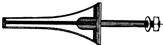
FIG. 105.—Solid metal pin.
