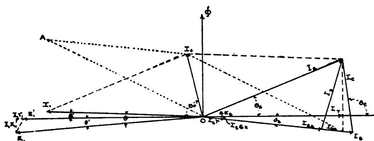
FIG. 7. HEYLAND MOTOR.
