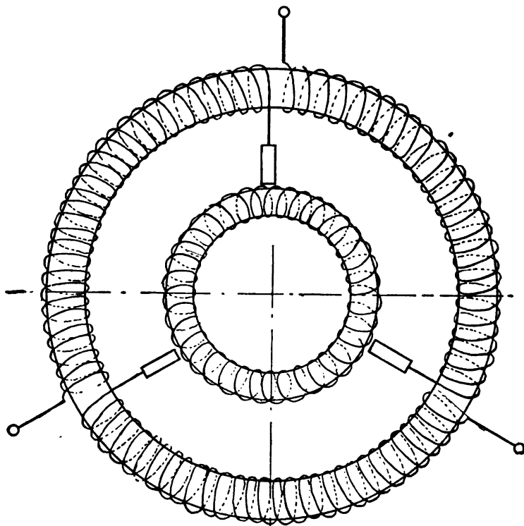
FIG. 1. GÖRGES MOTOR.
