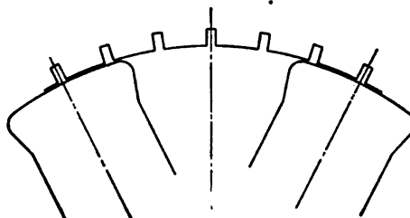
FIG. 15 360° = 1.25° 3 Slots per Pole
