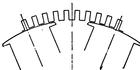
FIG. 13 360° = 1.25° 3 Slots per Pole
