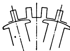
FIG. 14 360° = 1.25° 3 Slots per Pole
