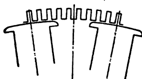
FIG. 11 360° = 1.25° 3 Slots per Pole
