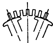
FIG. 10 360° = 1.25° 3 Slots per Pole
