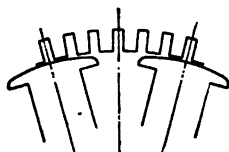
FIG. 12 360° = 1.25° 3 Slots per Pole
