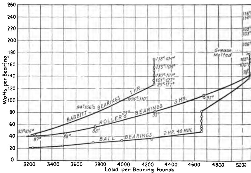
FIG. 27 BREAK DOWN TESTS, 200 R.P.M., 128 FT. PER MIN.
