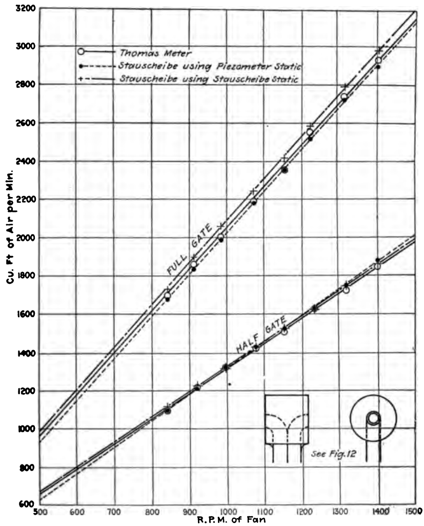
FIG. 25 STAUSCHEIBE S
