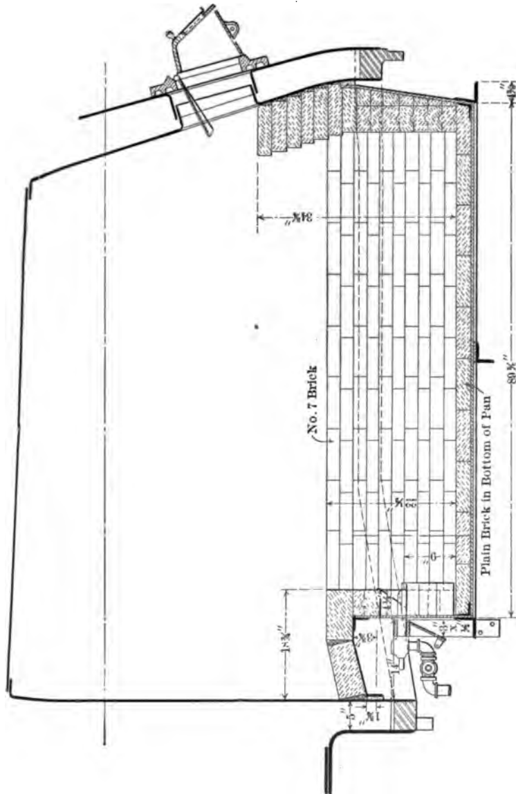
FIG. 3 LONGITUDINAL SECTION OF FIRE BOX
