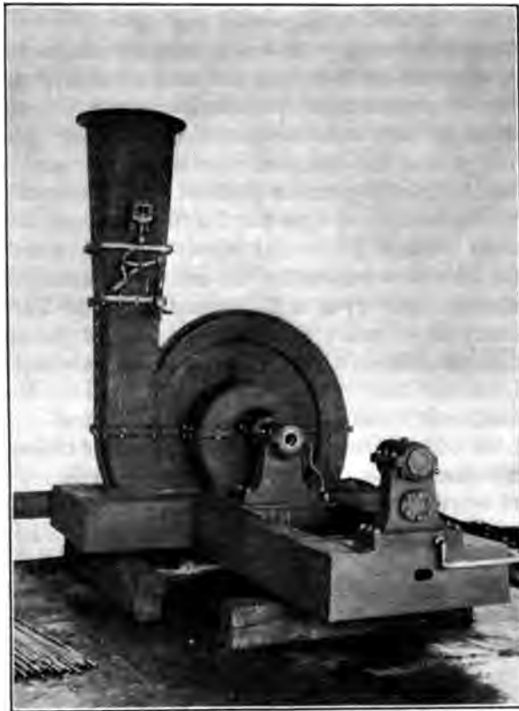
FIG. 9 A 600-H.P. BLOWER OF FREE-DIFFUSION TYPE
