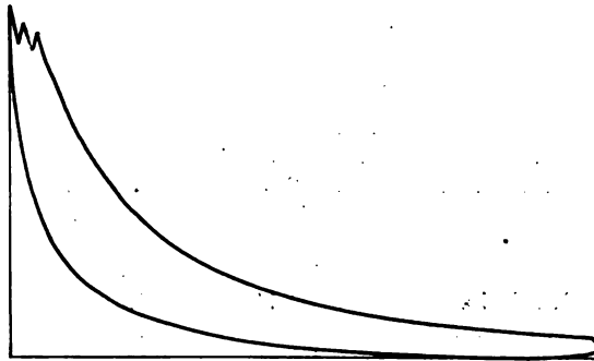
FIG. 41 TYPICAL INDICATOR DIAGRAM, TEST A 180 r.p.m.; 89 m.e.p.; 126 i.h.p.
