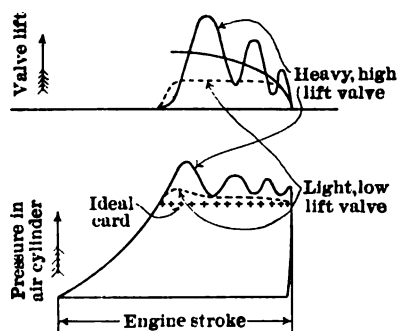
FIG. 4 ACTUAL MOTION OF OUTLET VALVES (DISPLACEMENT BASIS)
