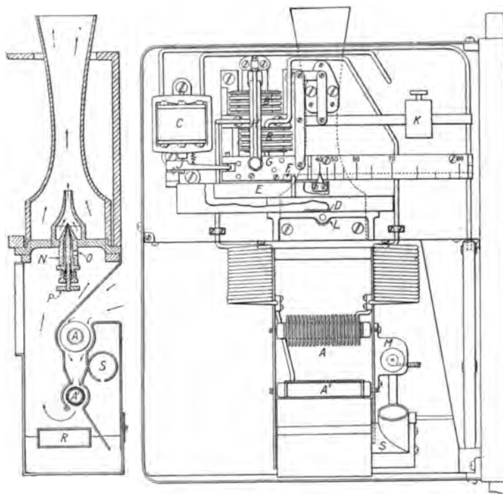
FIG. 22 VAPOR PRESSURE HYGROSTAT
