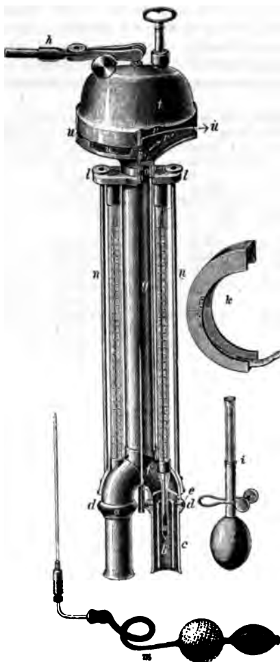
FIG. 11 ASPIRATION PSYCHROMETER
