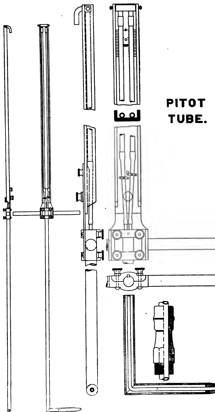
FIG. 8 PITOT TUBE
